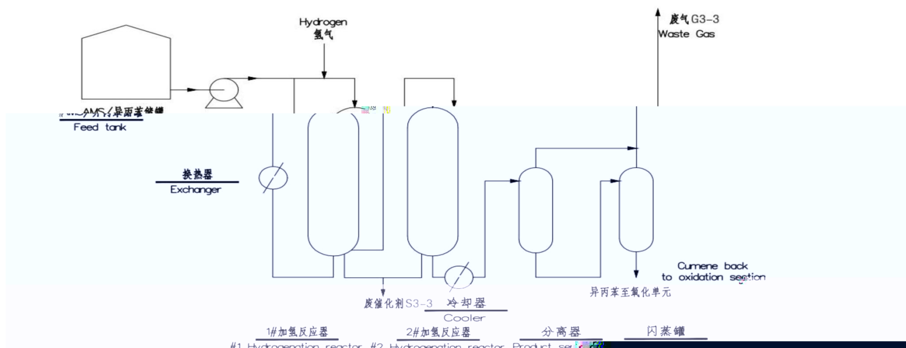
苯酚丙酮生产工艺流程及产污环节图（精馏提纯单元）
